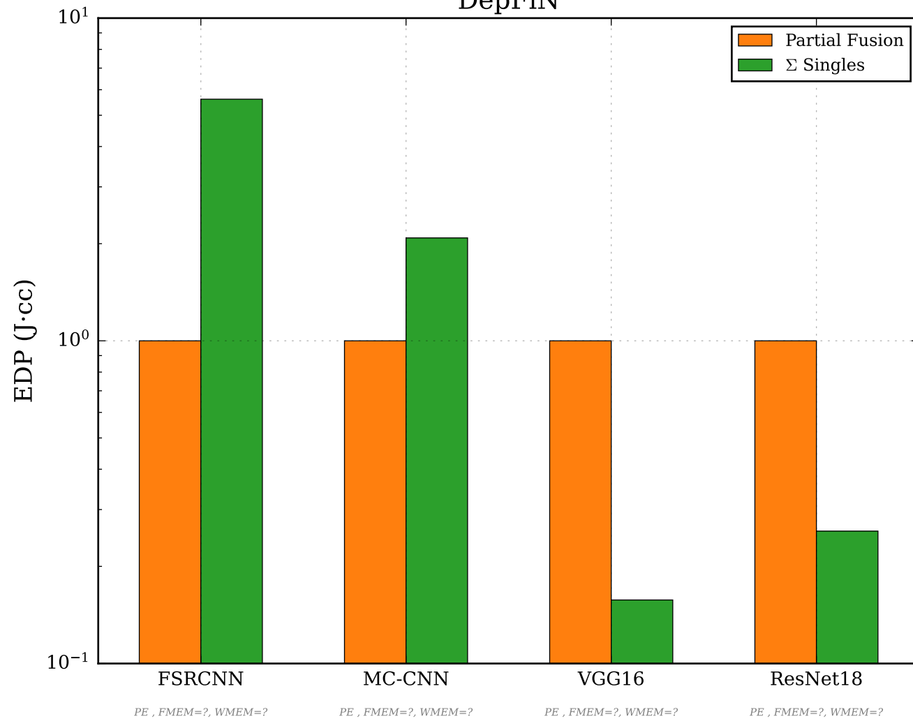
DepFiN
