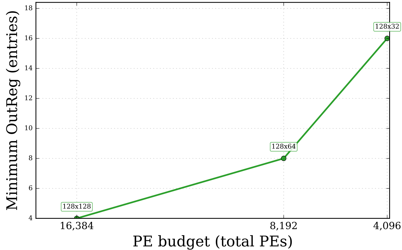
VGG16
