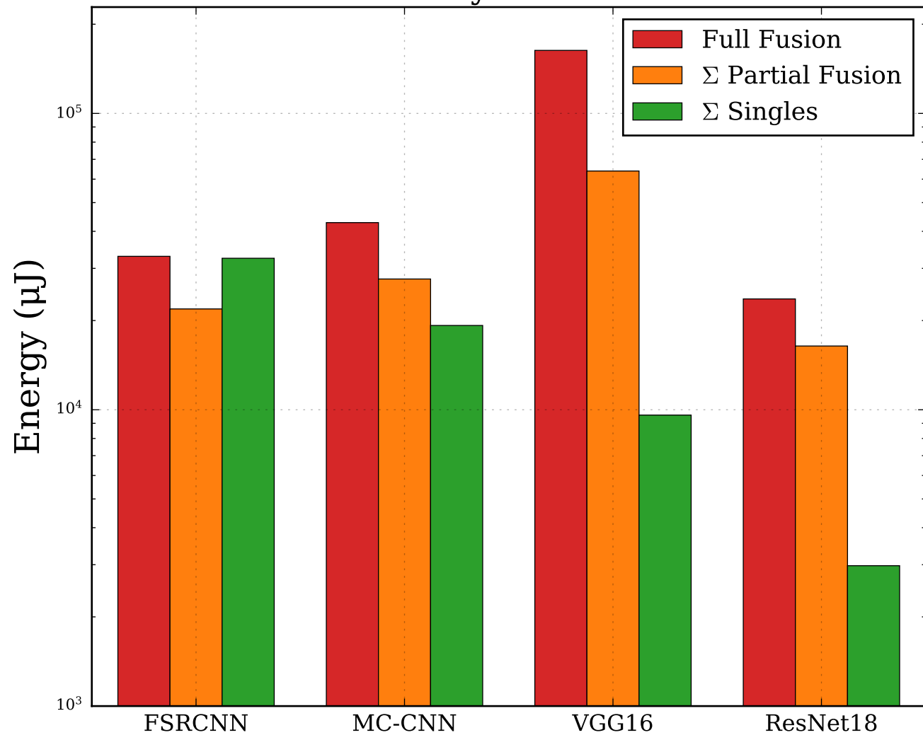
Eyeriss
