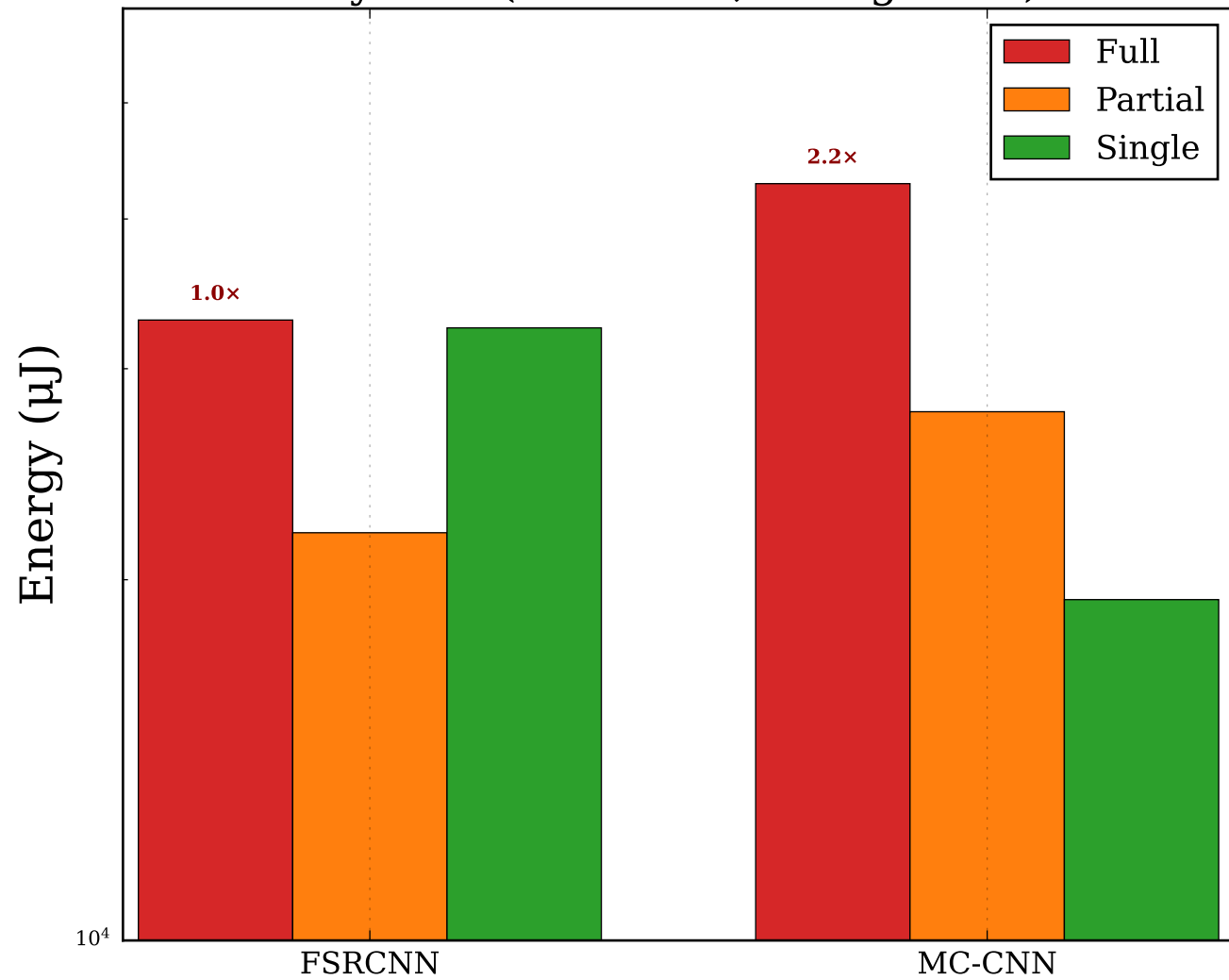
Eyeriss (2048 PEs, WReg=384)
