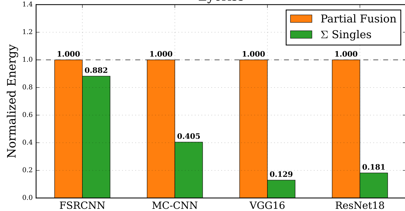
Eyeriss
