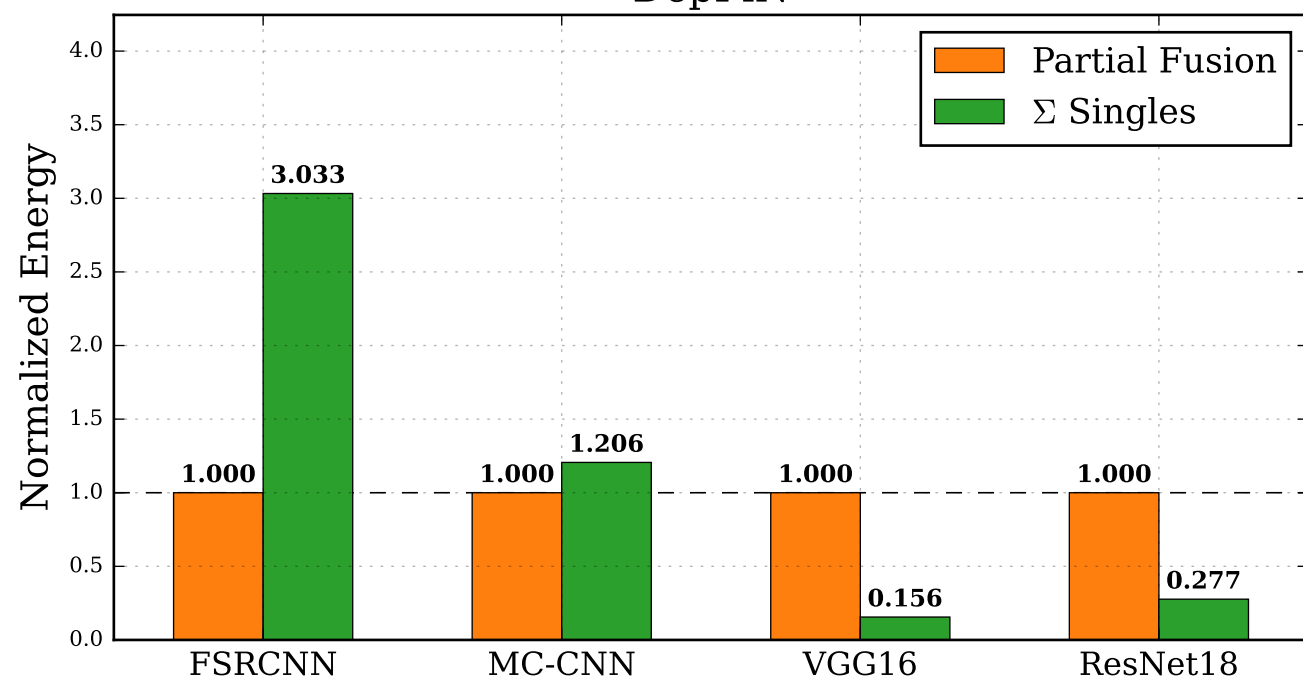
DepFiN
