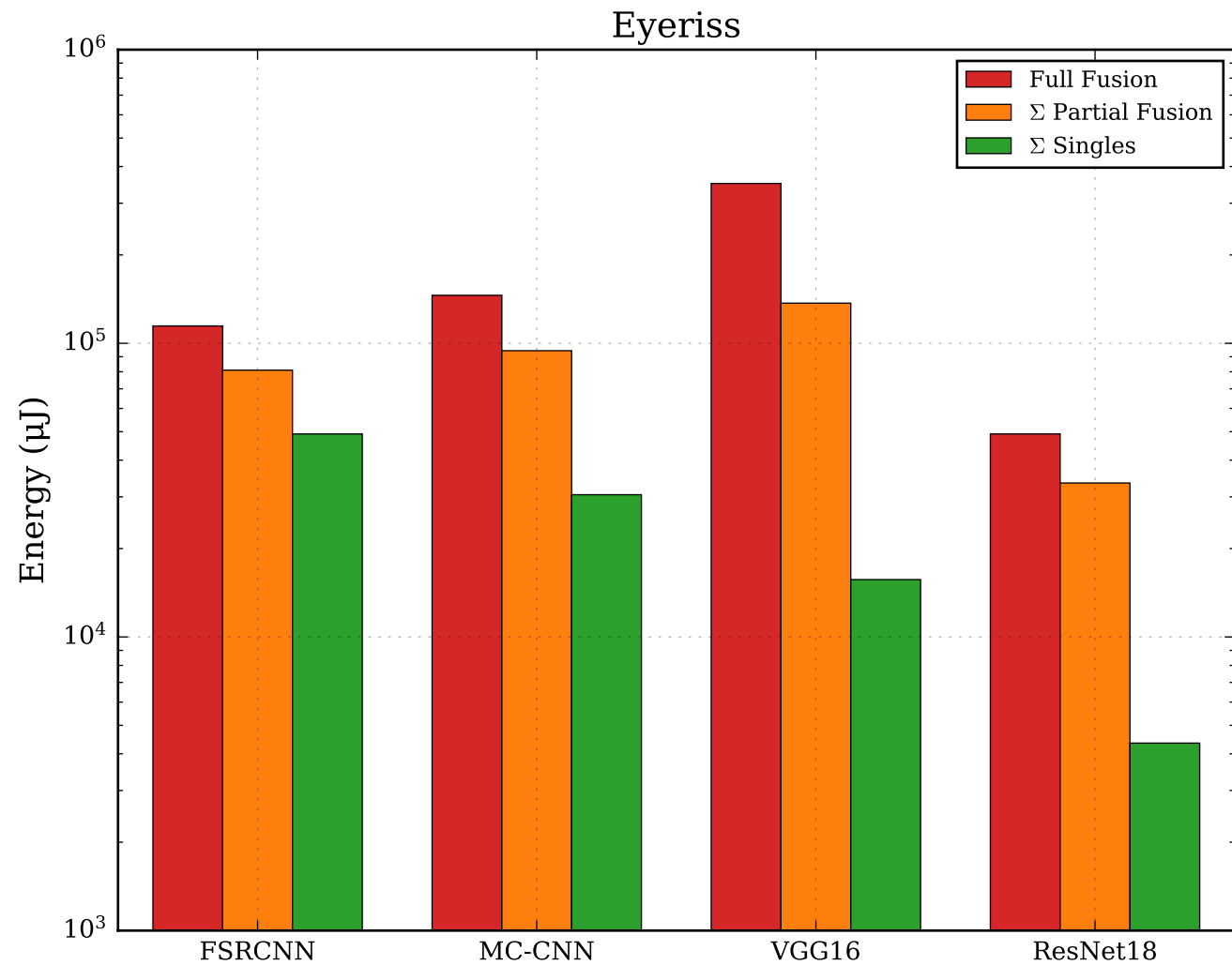
Scenario A — Energy (DRAM = 200 pJ/byte)
