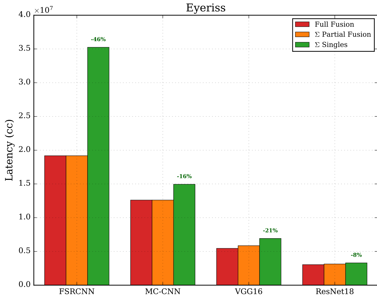
Scenario A — Latency (DRAM = 200 pJ/byte)
