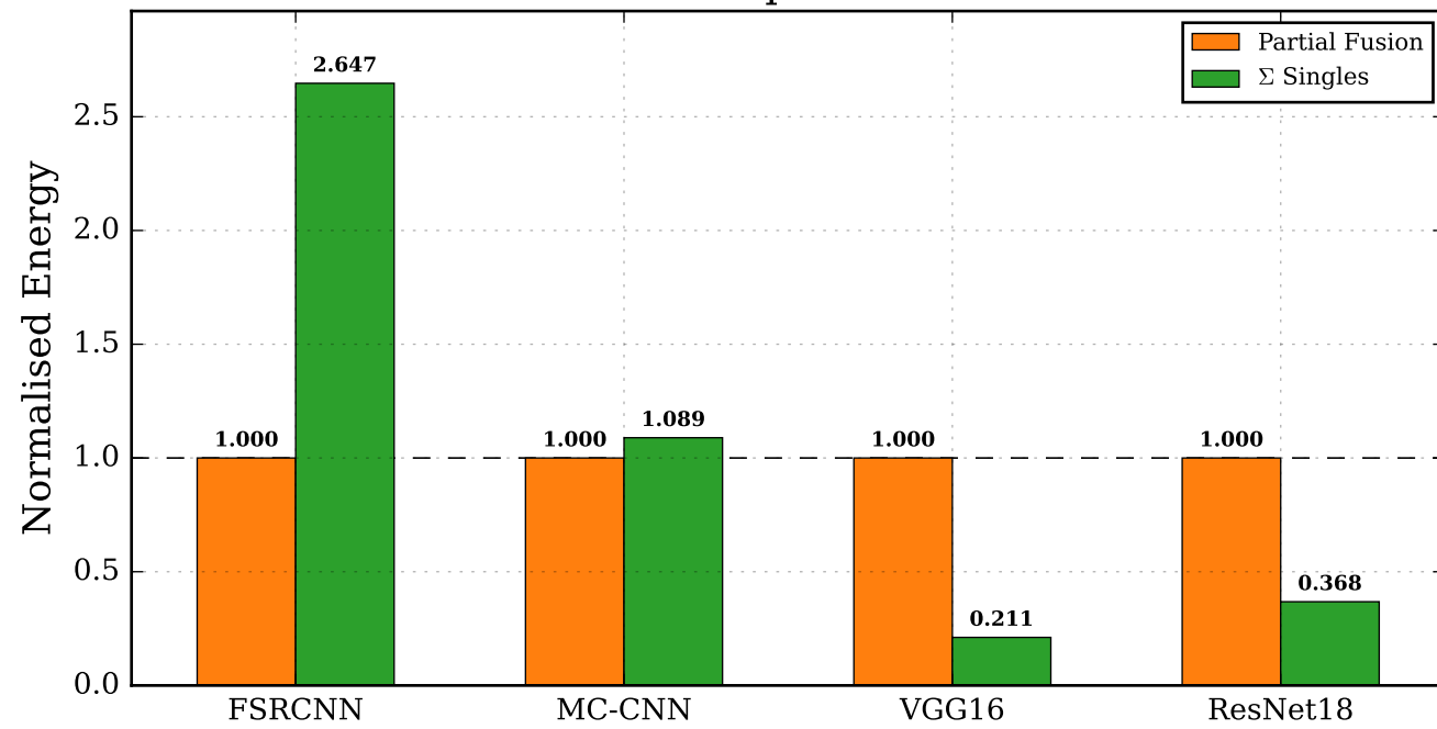
DepFiN
