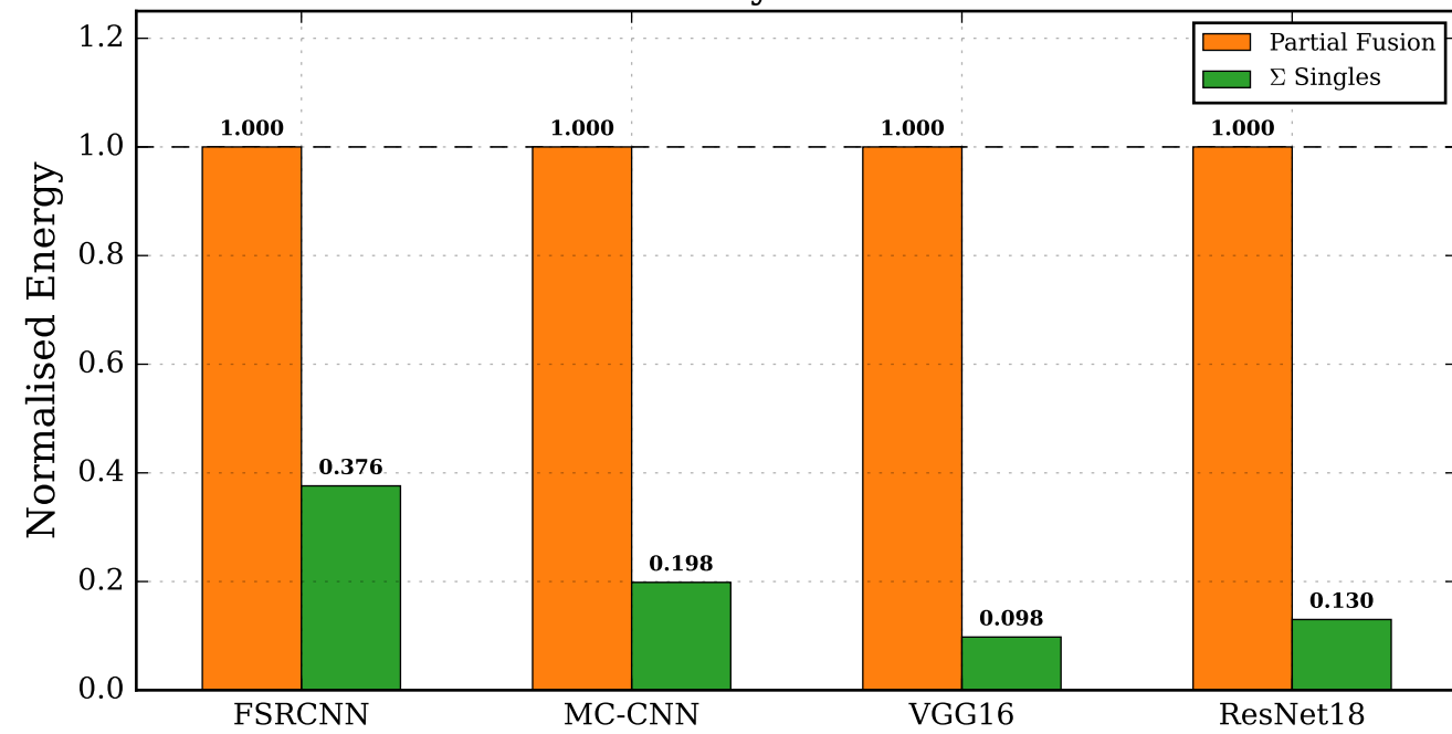
Eyeriss
