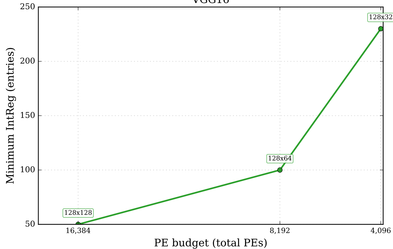
VGG16
