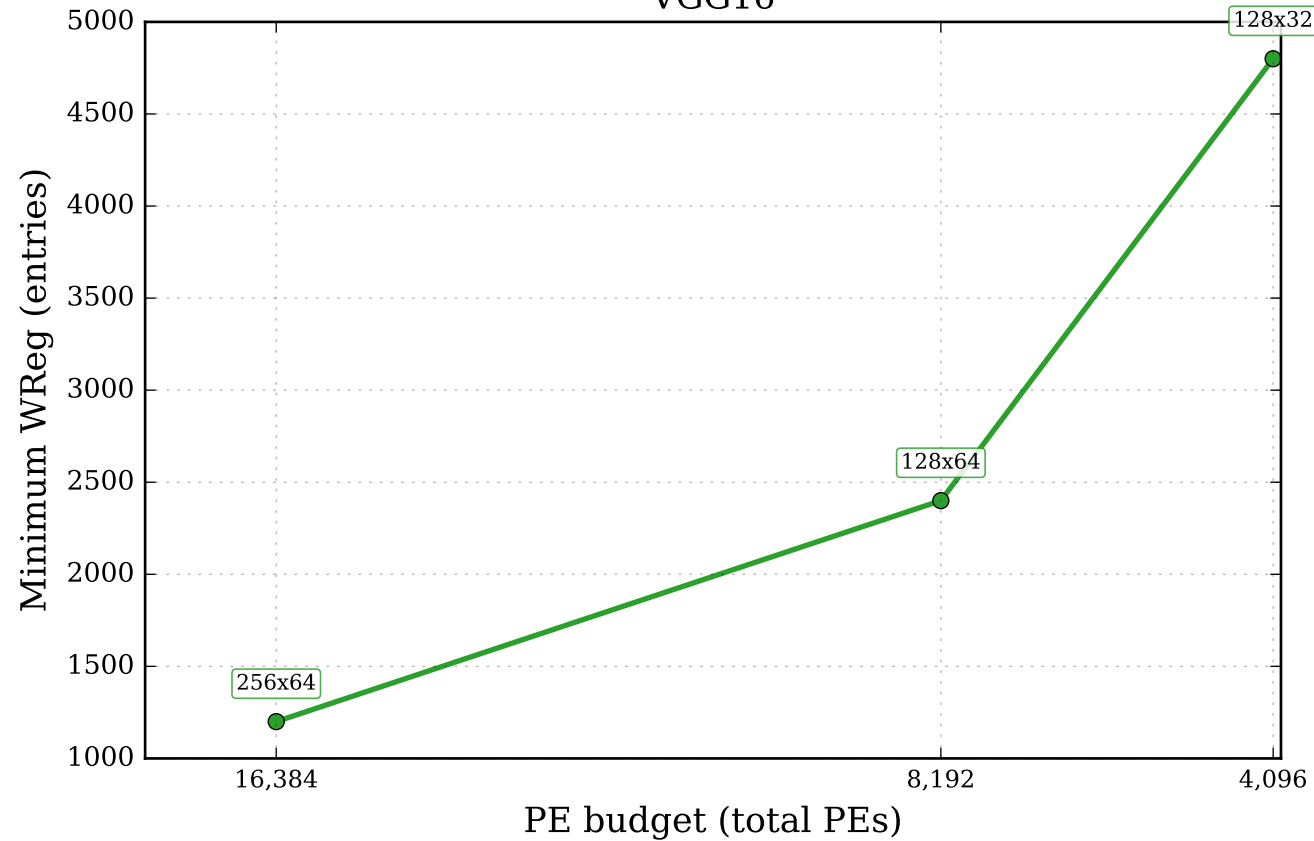
VGG16
