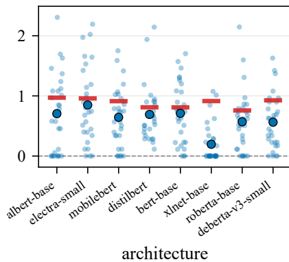
CoLA
