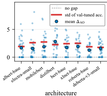
RTE
