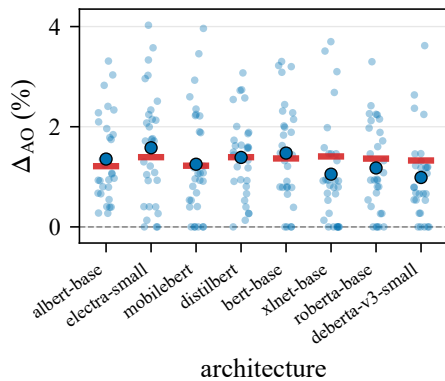
MRPC
