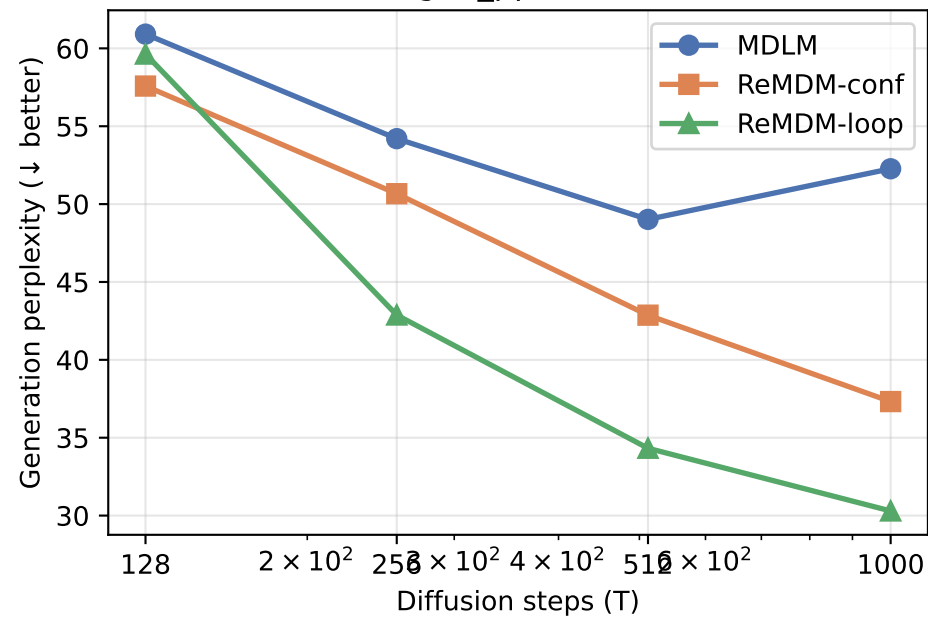
gen_ppl vs T
