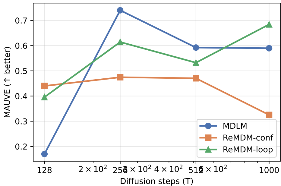
MAUVE vs T
