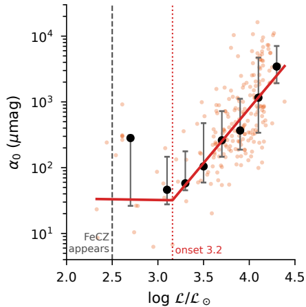
c \alpha_0 , OB stars (N=222)
