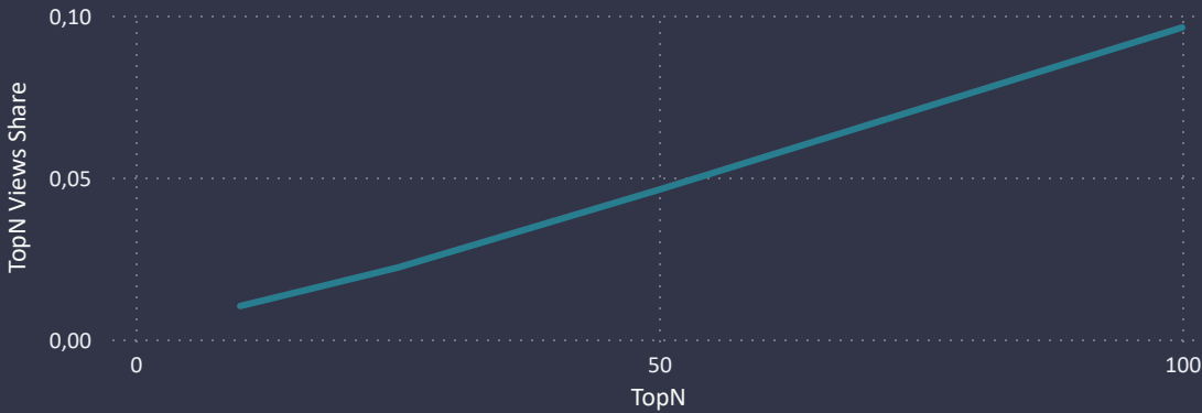
TopN Views Share by TopN
