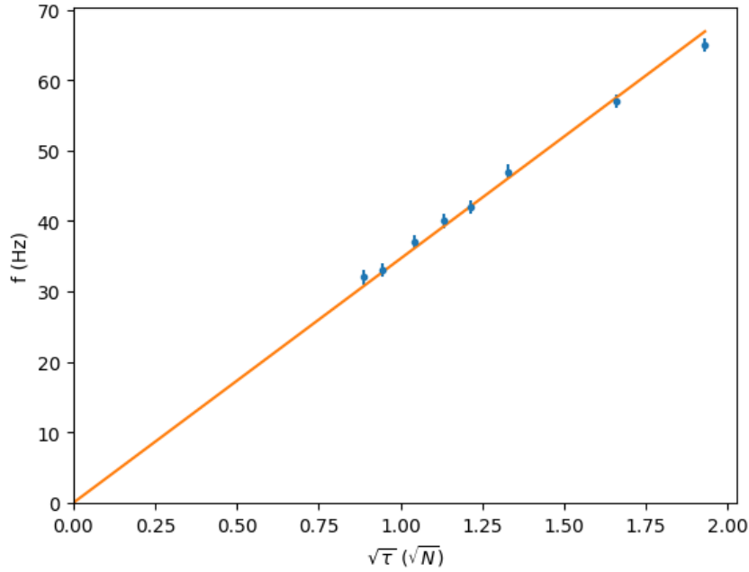
Figura 2: Dipendenza della frequenza dalla radice quadrata della tensione applicata alla corda.
