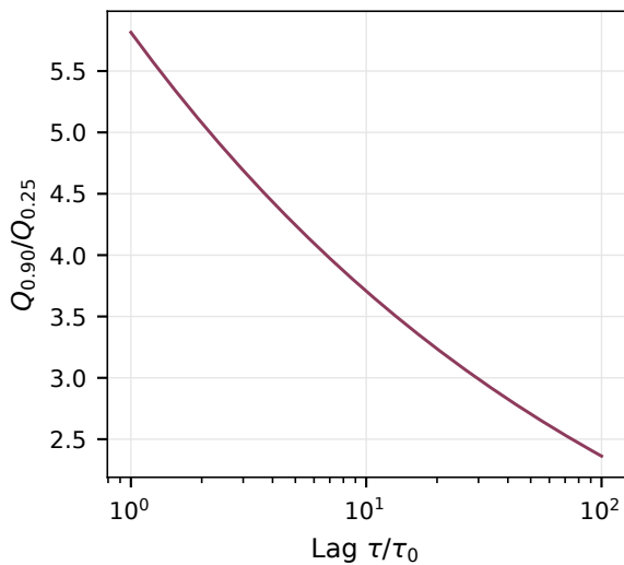
(d) Quantile ratio
