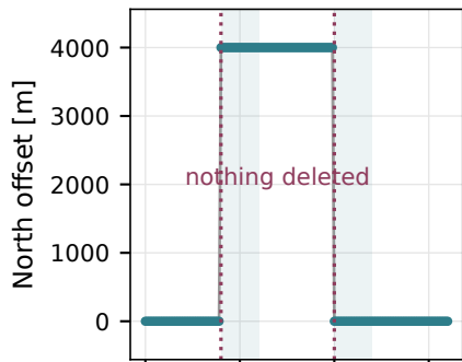
(f) No rejoin in w : cut
