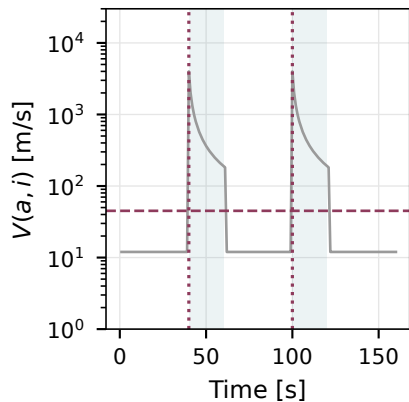
(f) No rejoin in w : cut
