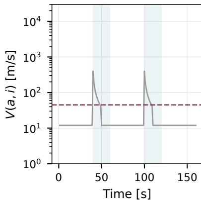
(d) Rejoins in w : deleted
