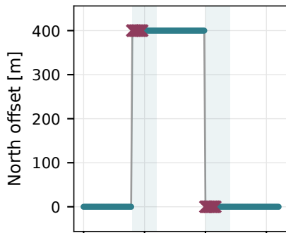
(d) Rejoins in w : deleted
