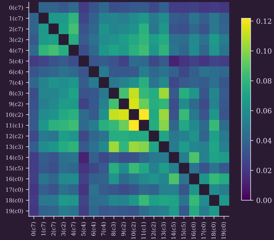
Edge Jaccard (max off-diag = 0.12)
