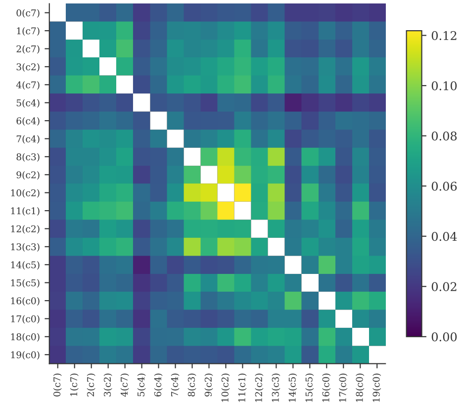
Edge Jaccard (max off-diag = 0.12)
