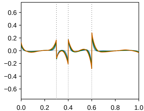
MLE
