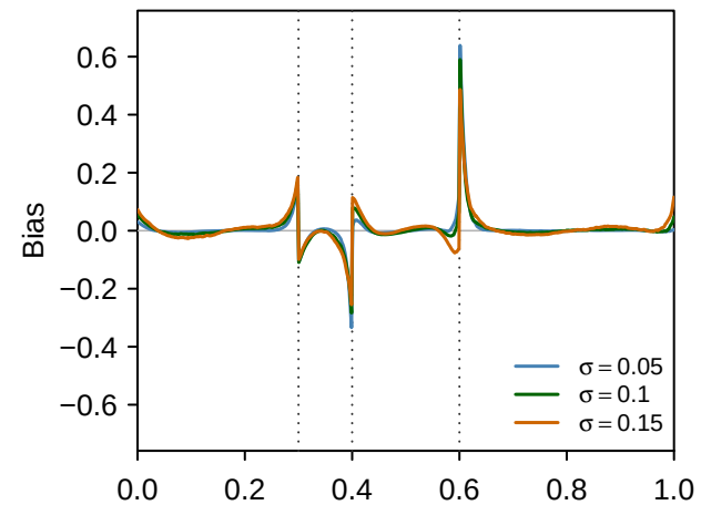
CSSD (CV)
