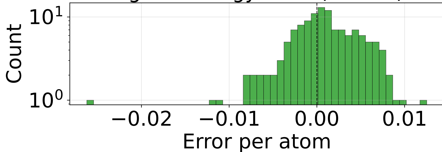
RMSE_E_per_atom (n=133)
