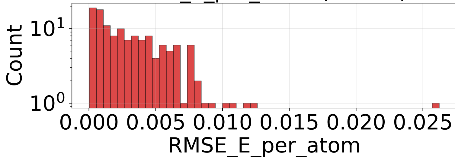
RMSE_E_per_atom (n=133)
