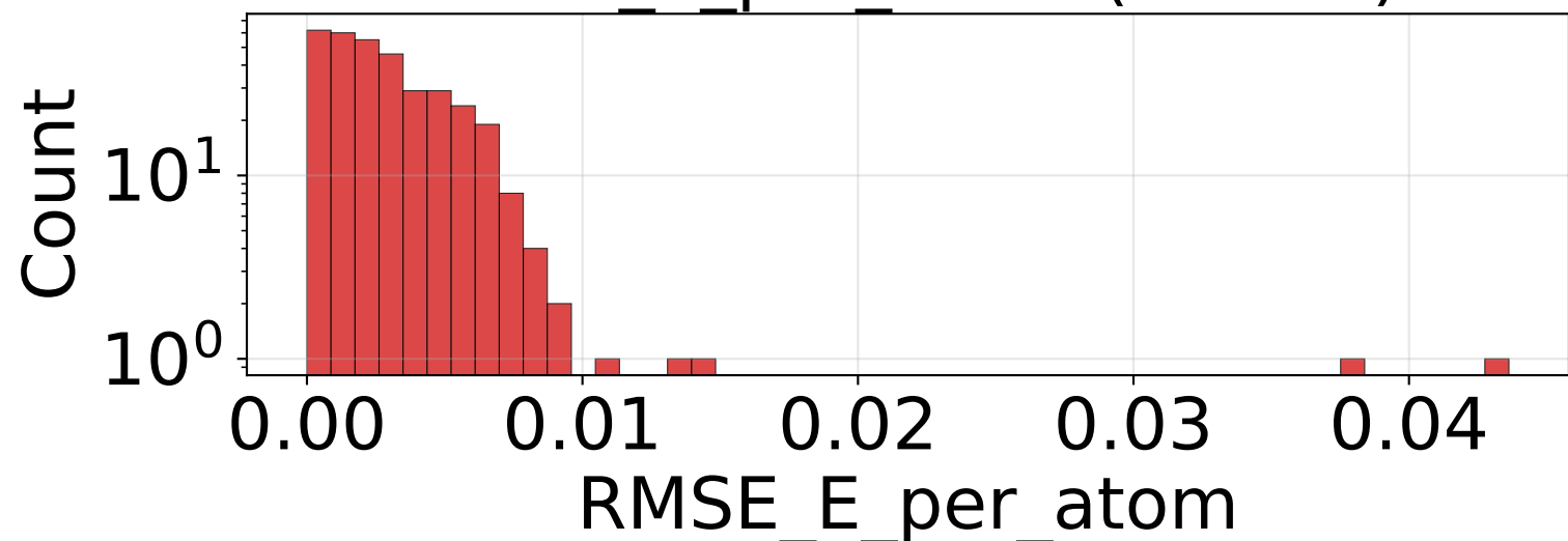
RMSE_E_per_atom (n=343)
