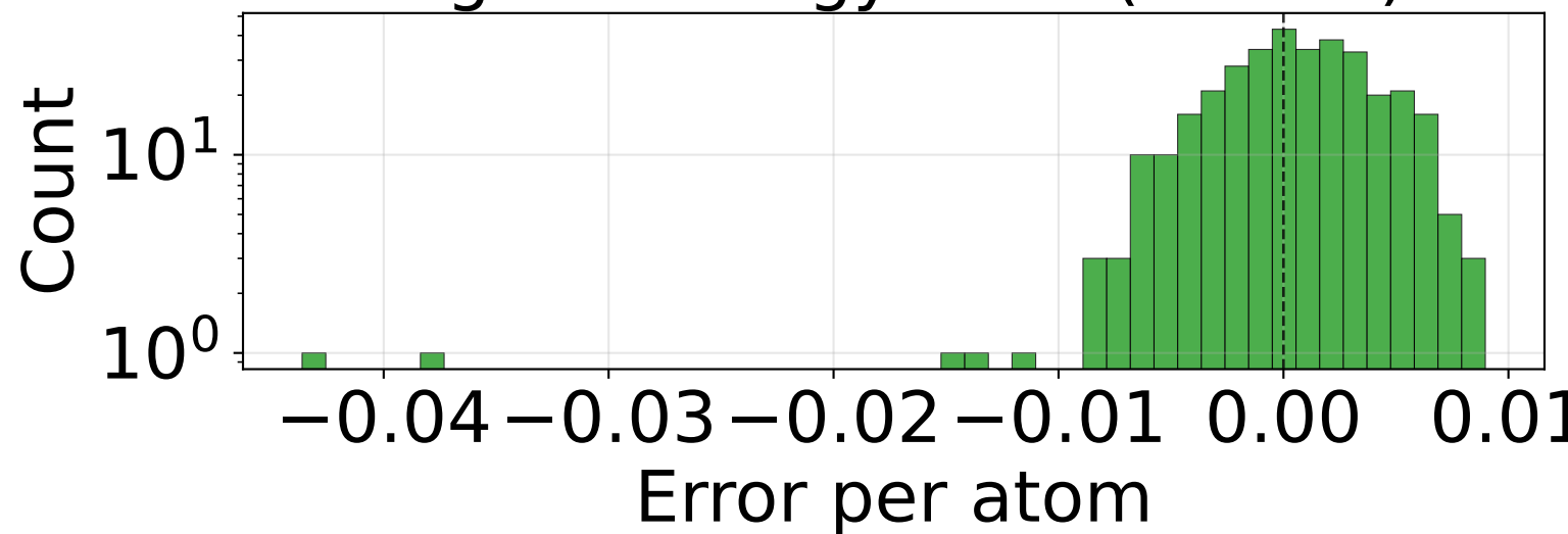
RMSE_E_per_atom (n=343)
