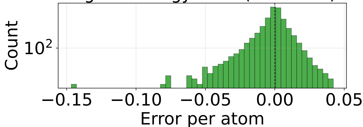
RMSE_E_per_atom (n=49500)
