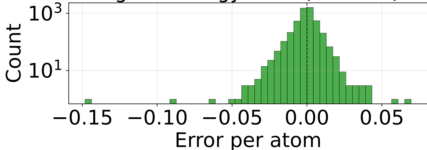
RMSE_E_per_atom (n=4950)
