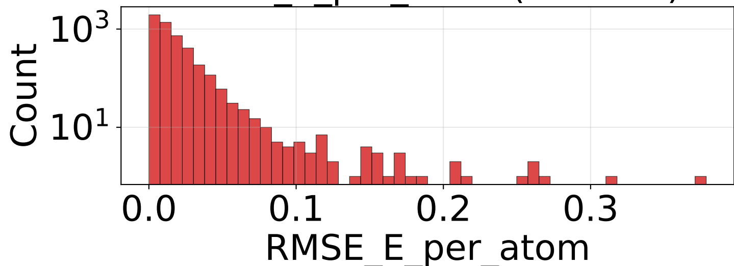
RMSE_E_per_atom (n=4950)
