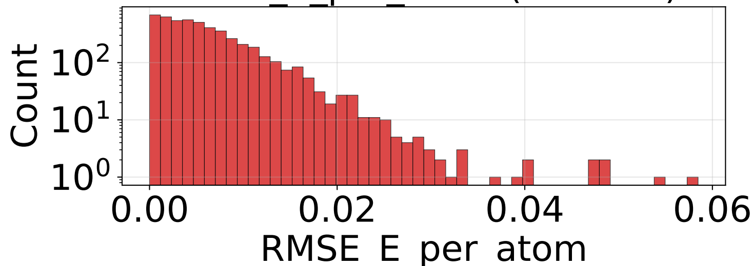
RMSE_E_per_atom (n=4950)
