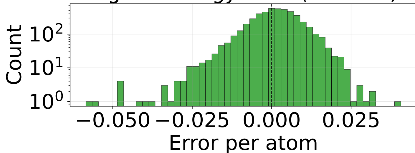
RMSE_E_per_atom (n=4950)
