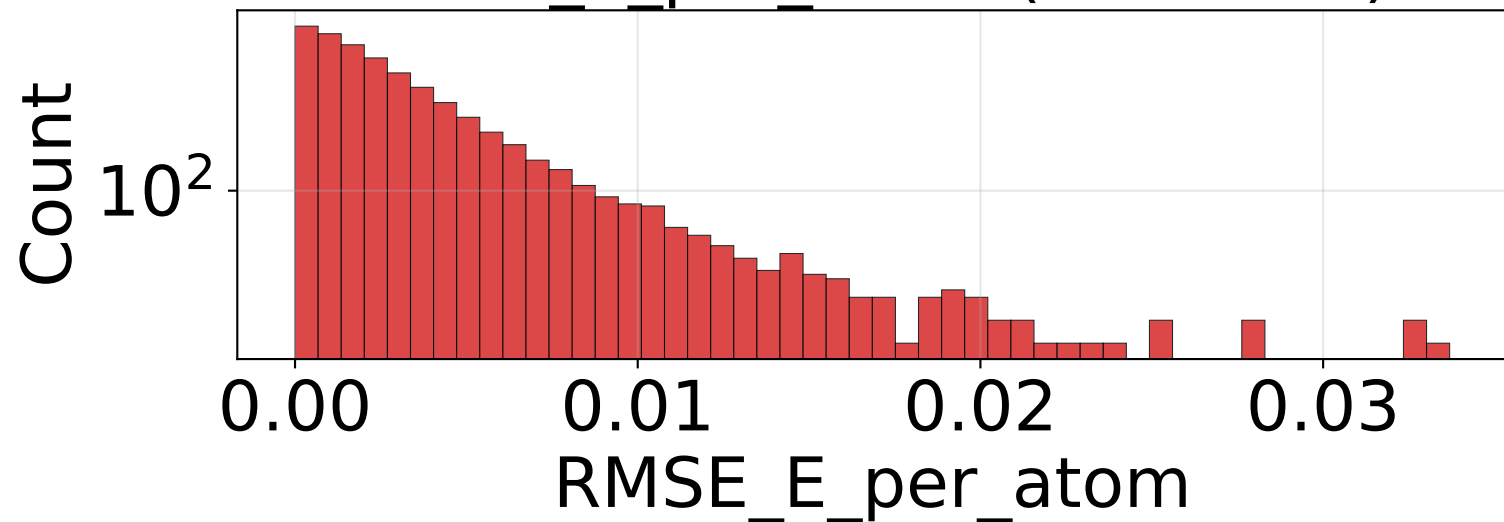
RMSE_E_per_atom (n=49500)
