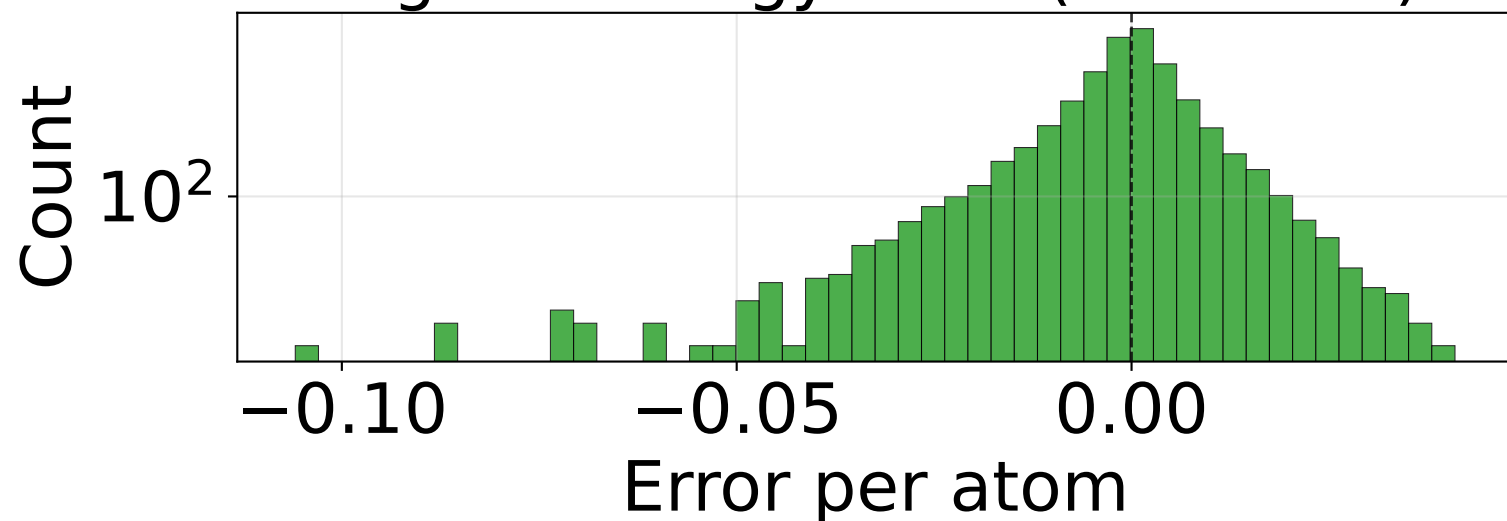
RMSE_E_per_atom (n=49500)
