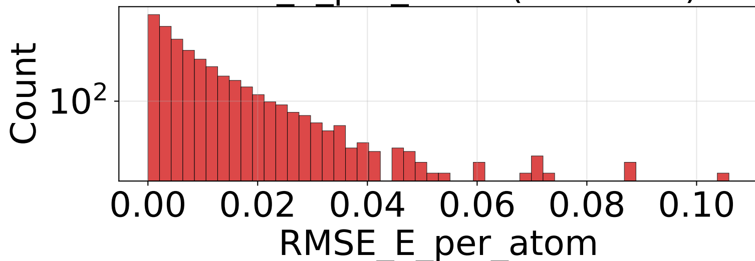
RMSE_E_per_atom (n=49500)
