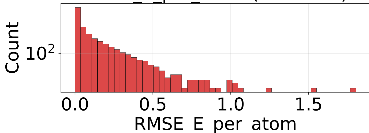
RMSE_E_per_atom (n=49500)
