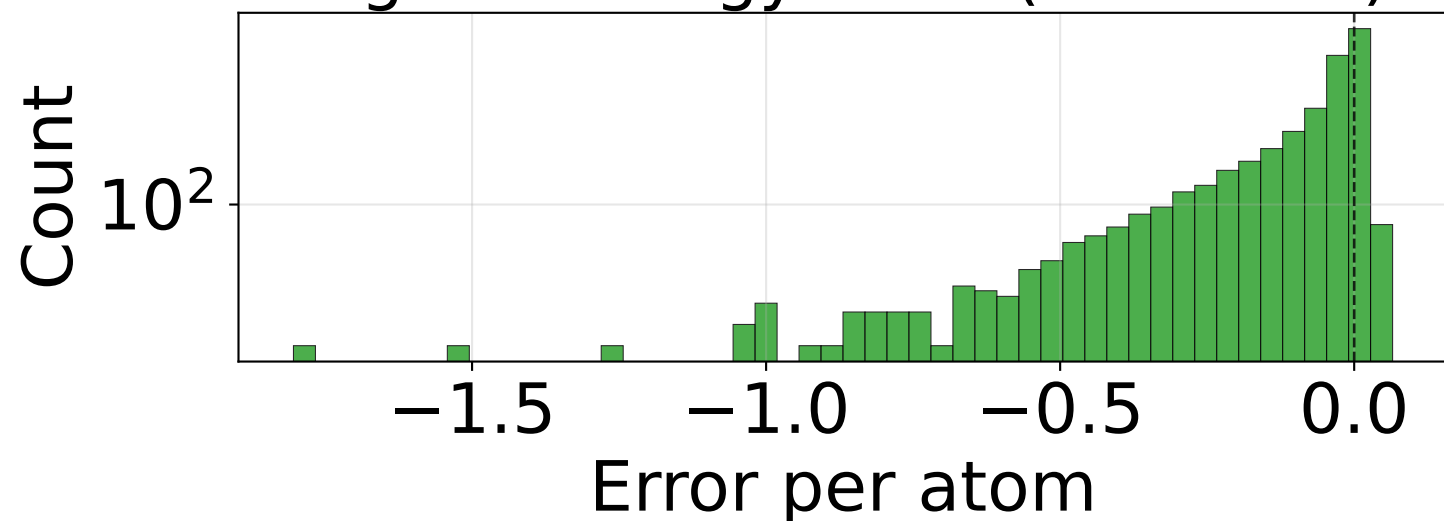
RMSE_E_per_atom (n=49500)
