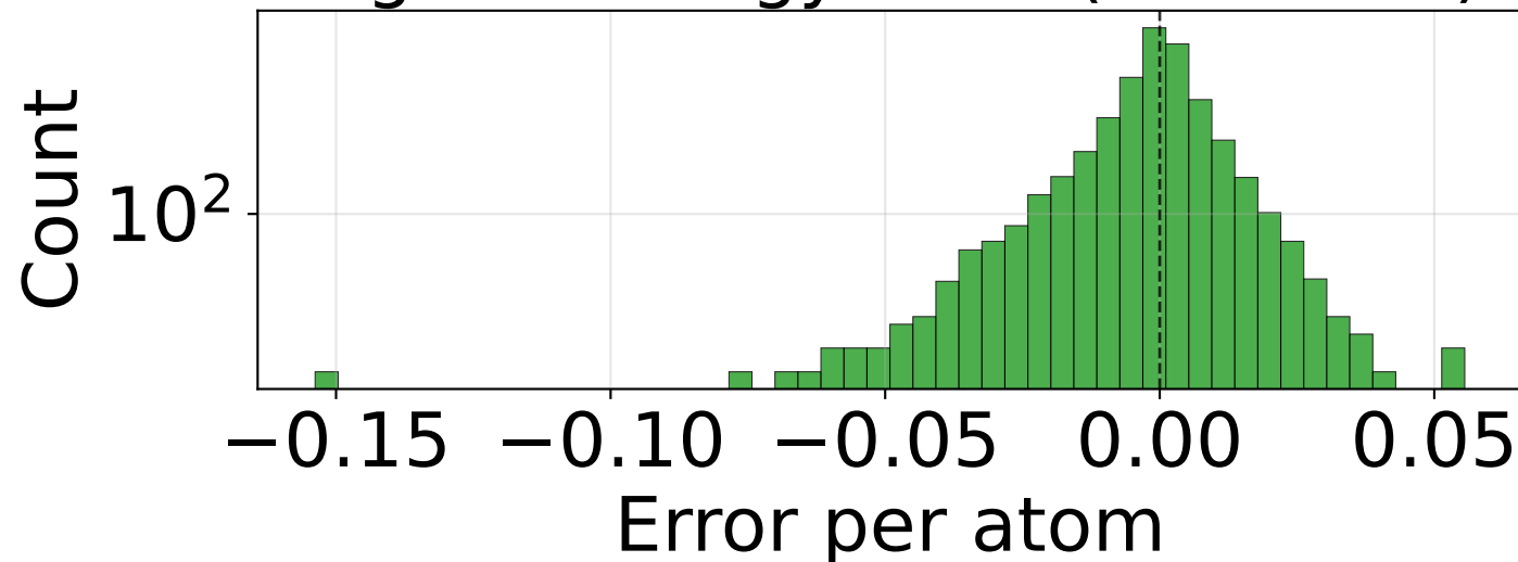
RMSE_E_per_atom (n=49500)
