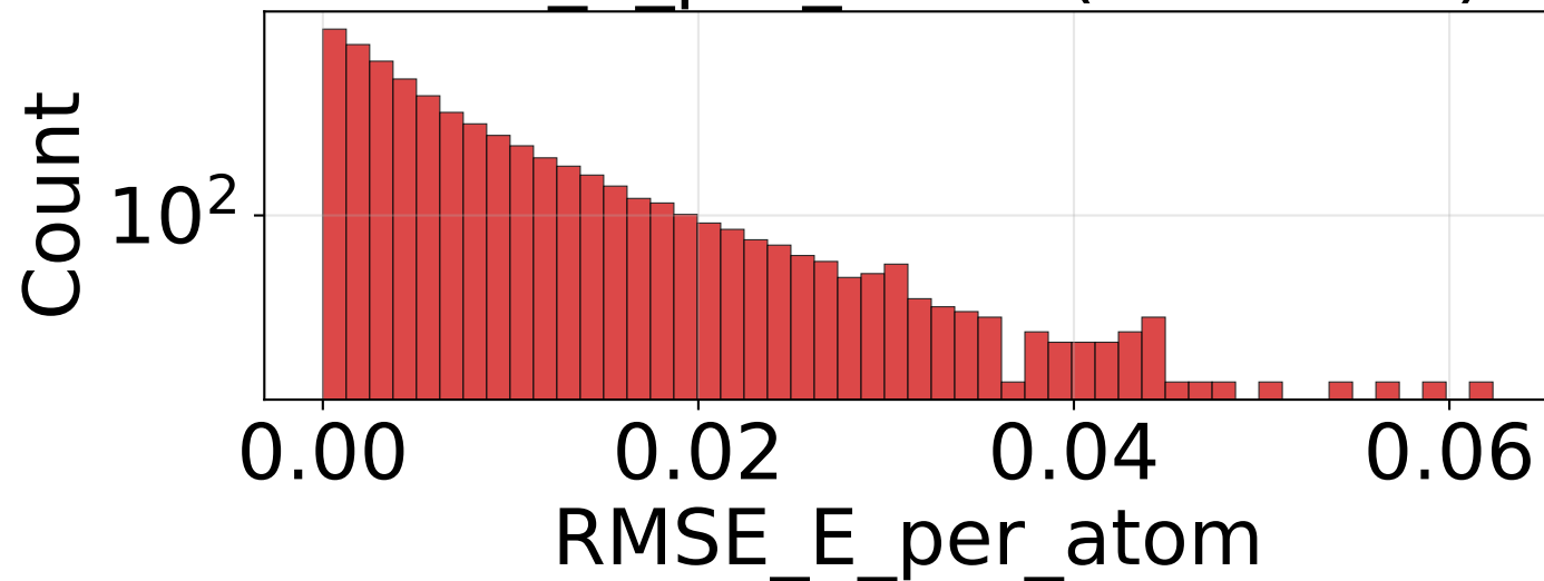
RMSE_E_per_atom (n=49500)
