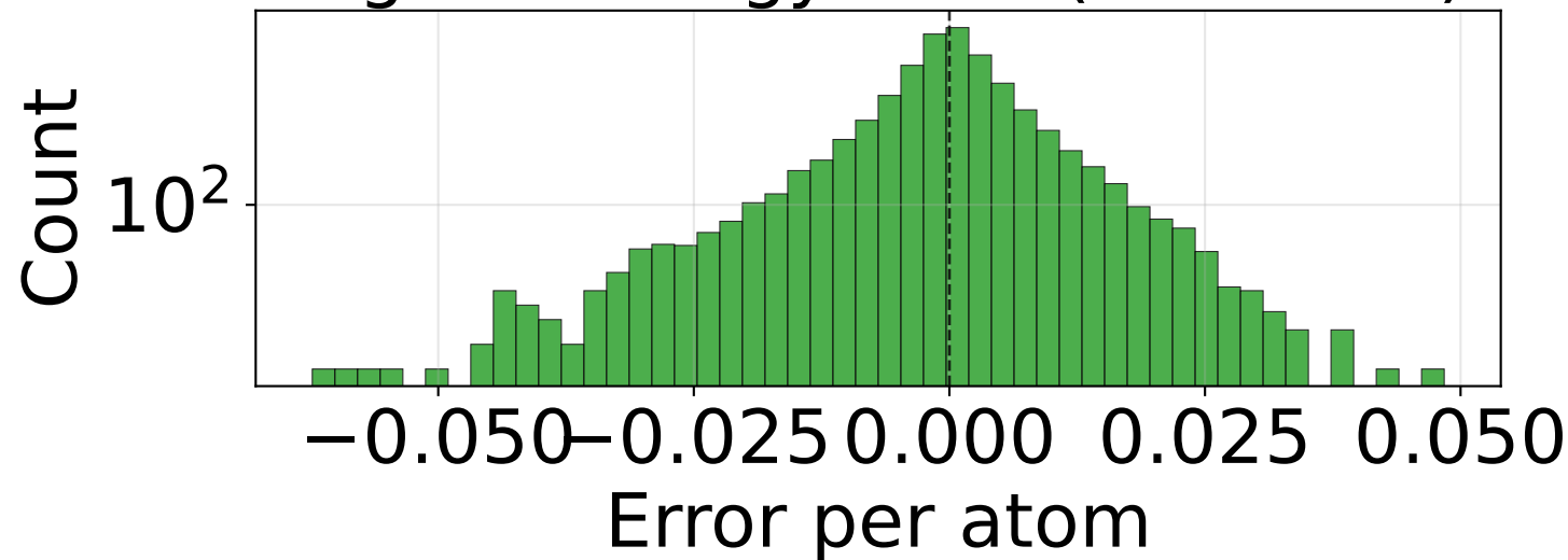
RMSE_E_per_atom (n=49500)
