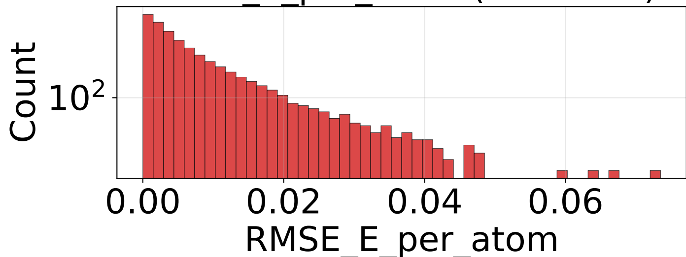
RMSE_E_per_atom (n=49500)
