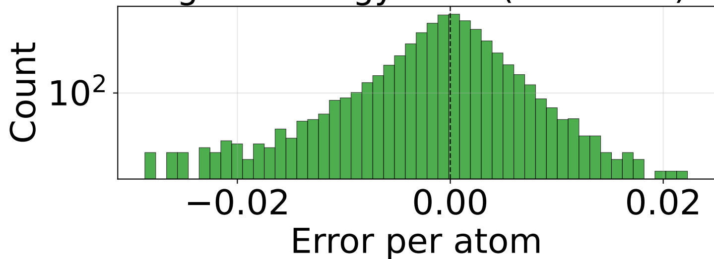
RMSE_E_per_atom (n=49500)
