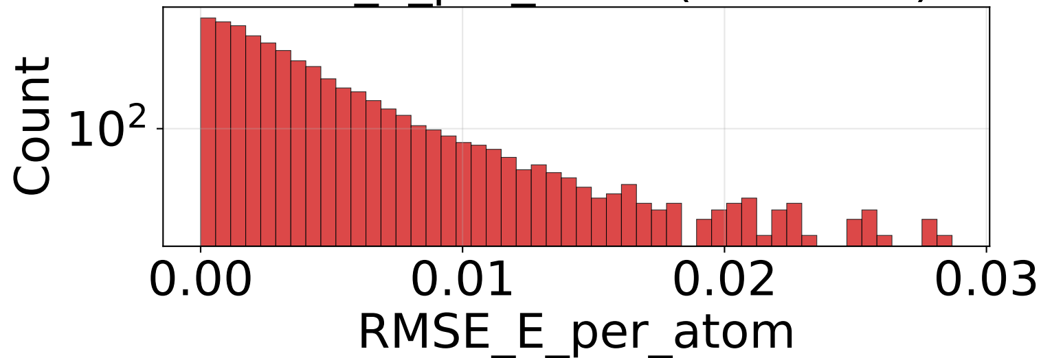
RMSE_E_per_atom (n=49500)
