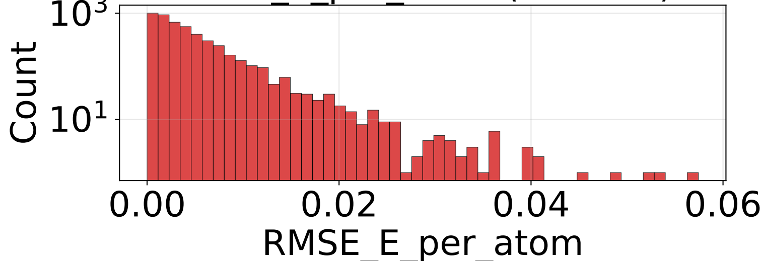
RMSE_E_per_atom (n=4950)
