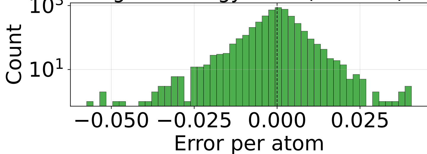
RMSE_E_per_atom (n=4950)
