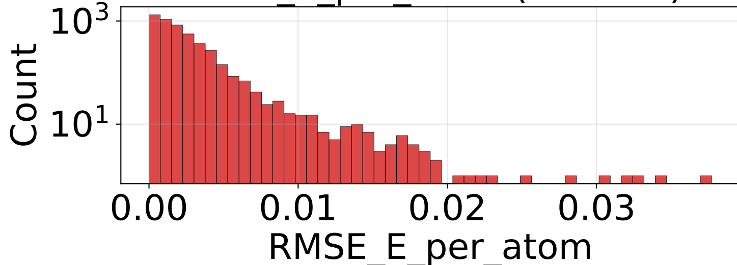
RMSE_E_per_atom (n=4950)
