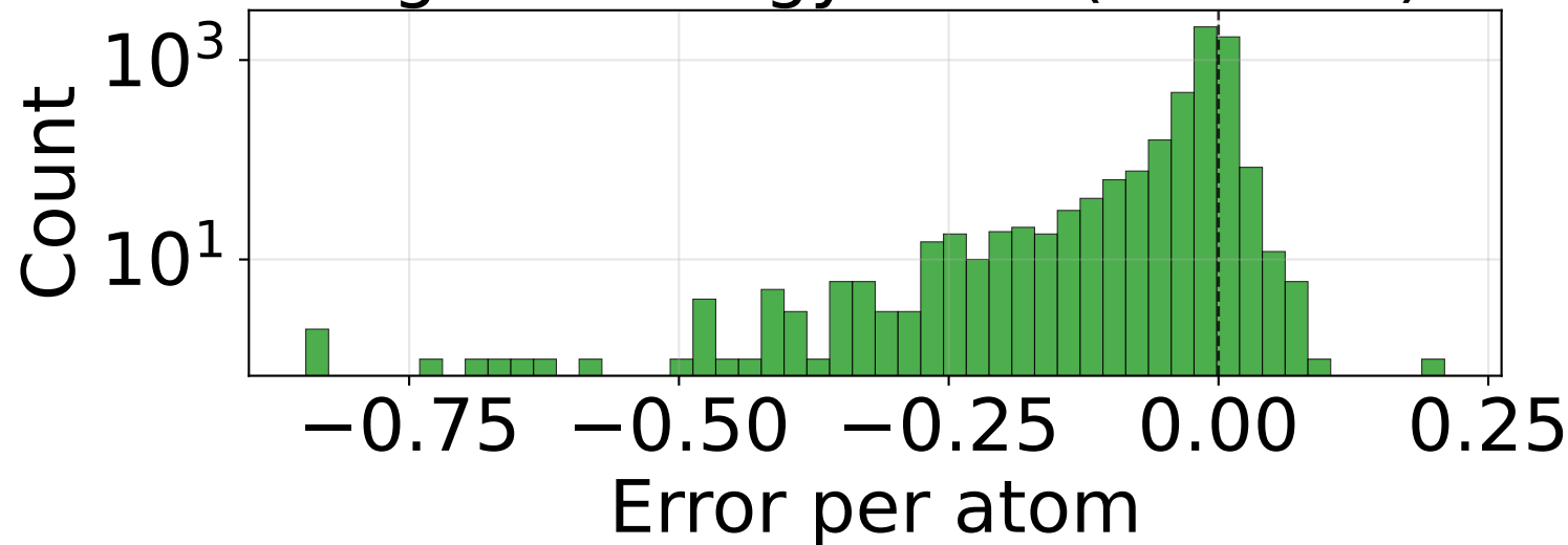
RMSE_E_per_atom (n=4950)
