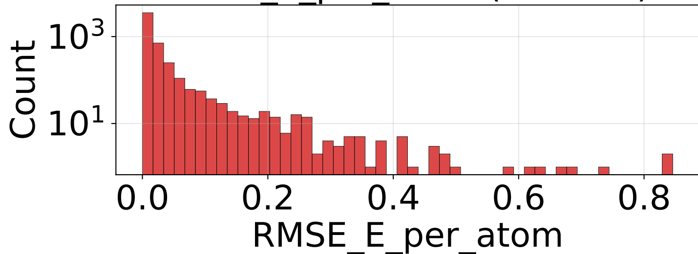
RMSE_E_per_atom (n=4950)
