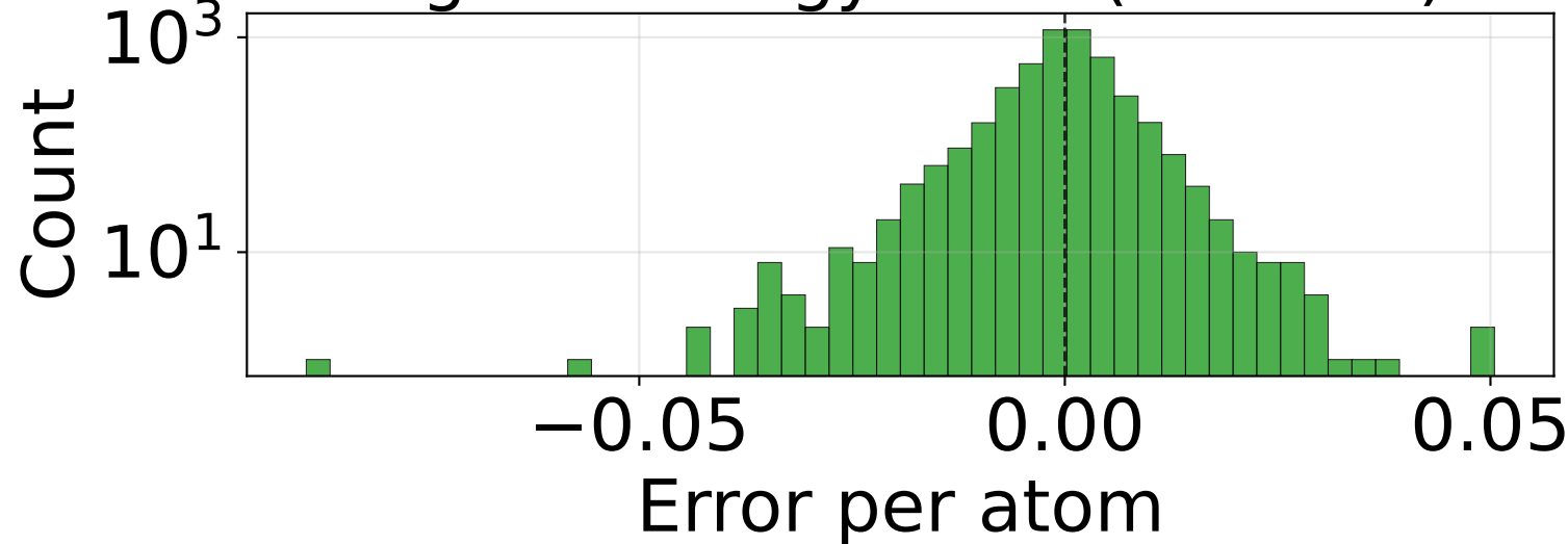
RMSE_E_per_atom (n=4950)
