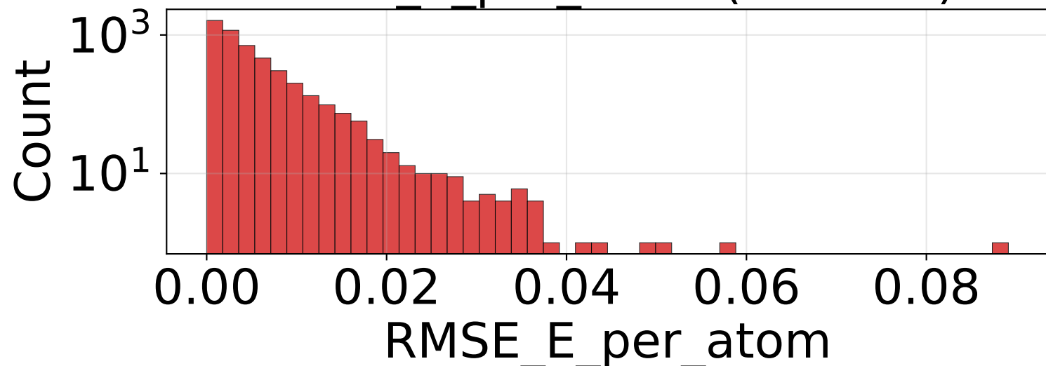
RMSE_E_per_atom (n=4950)
