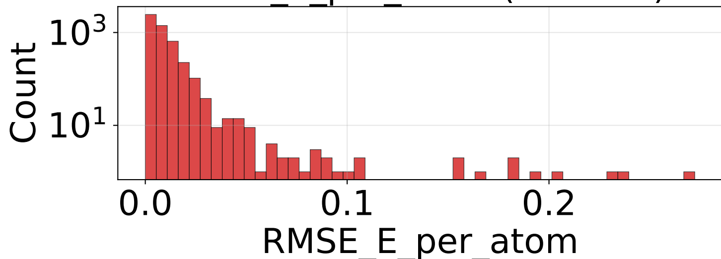
RMSE_E_per_atom (n=4950)
