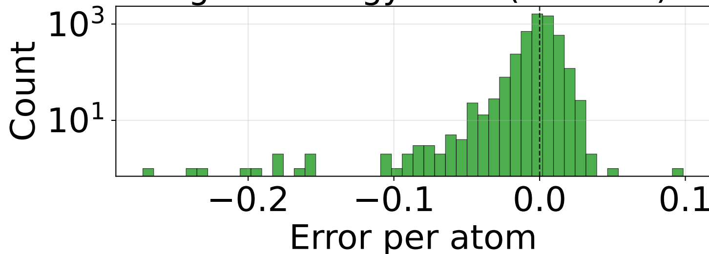
RMSE_E_per_atom (n=4950)
