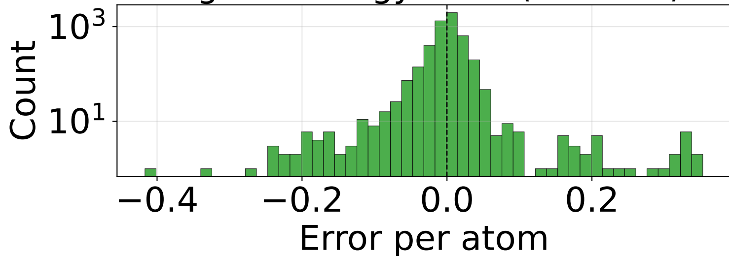
RMSE_E_per_atom (n=4950)
