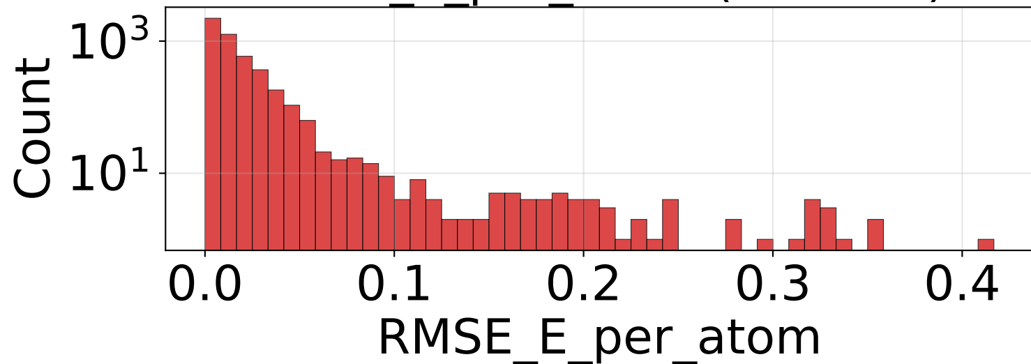
RMSE_E_per_atom (n=4950)
