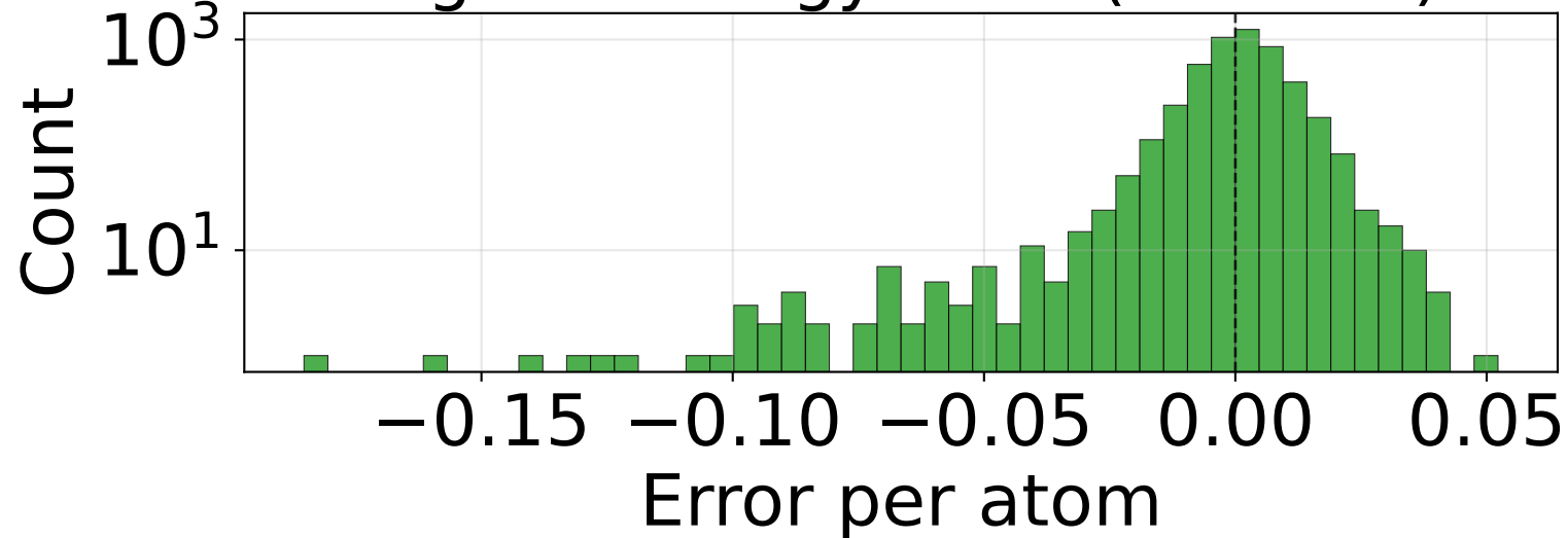
RMSE_E_per_atom (n=4950)
