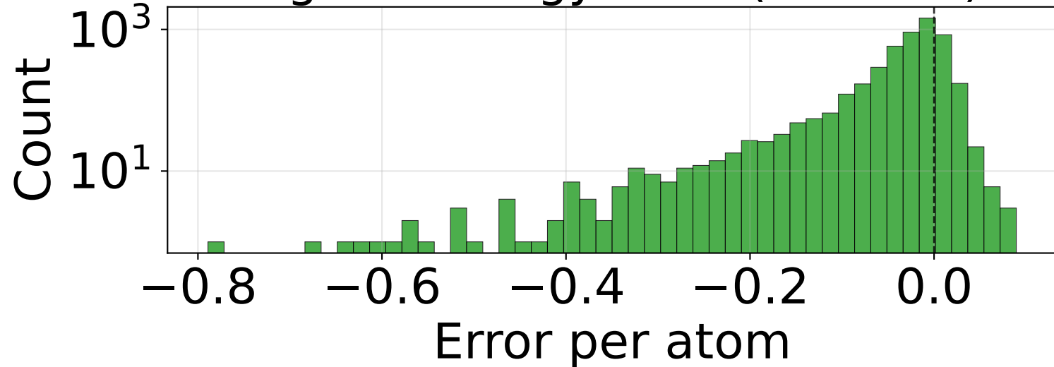
RMSE_E_per_atom (n=4950)
