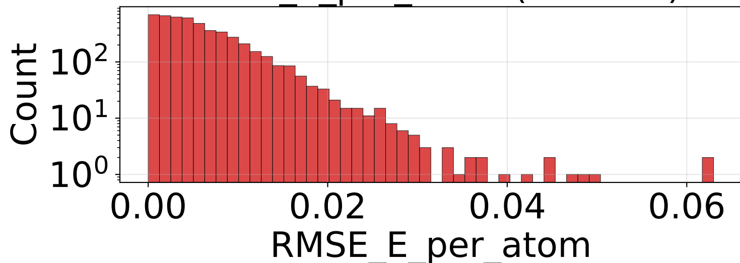
RMSE_E_per_atom (n=4950)
