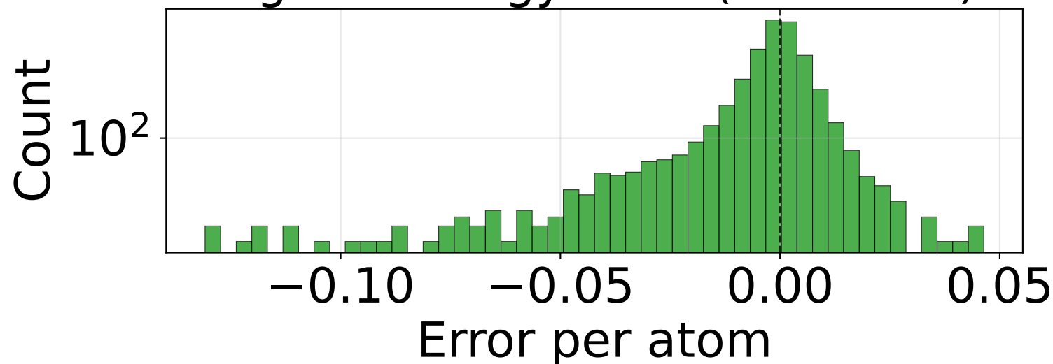
RMSE_E_per_atom (n=49500)
