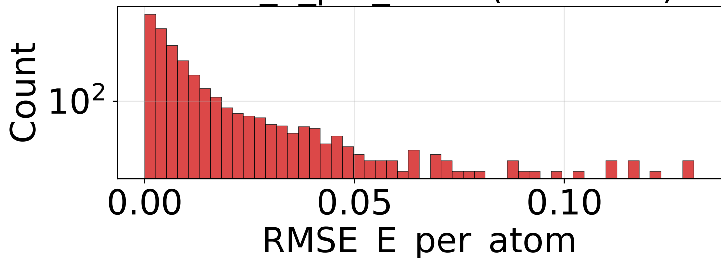
RMSE_E_per_atom (n=49500)
