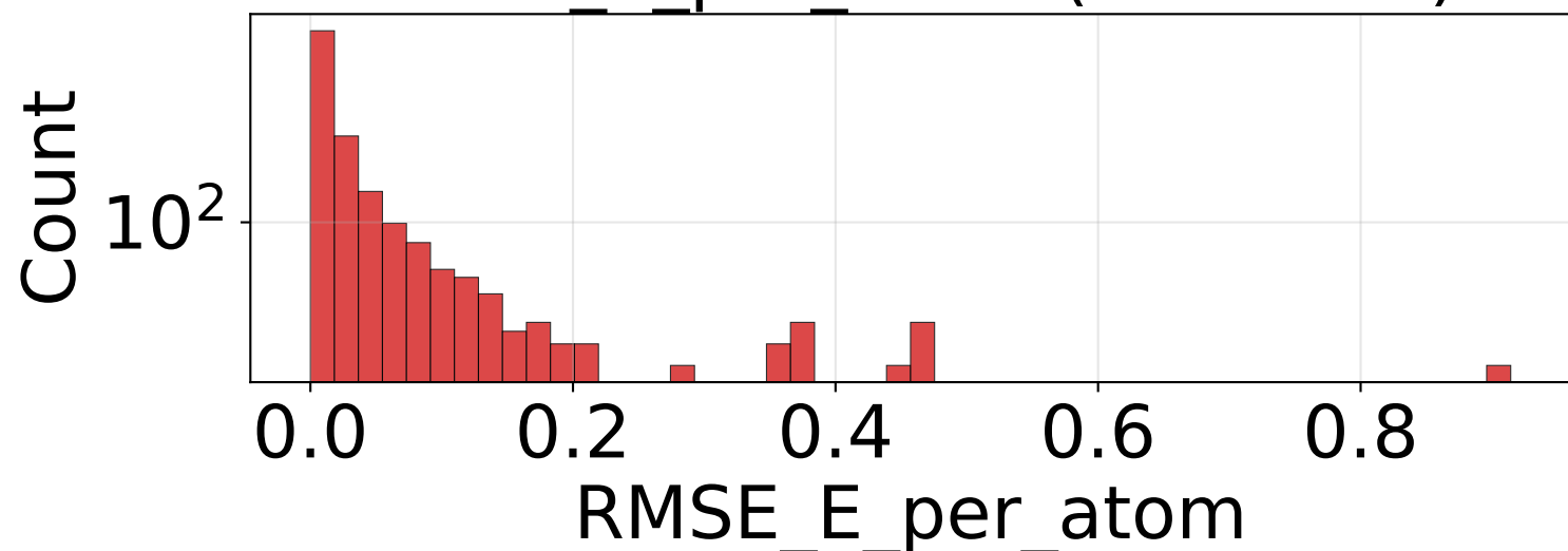
RMSE_E_per_atom (n=49500)
