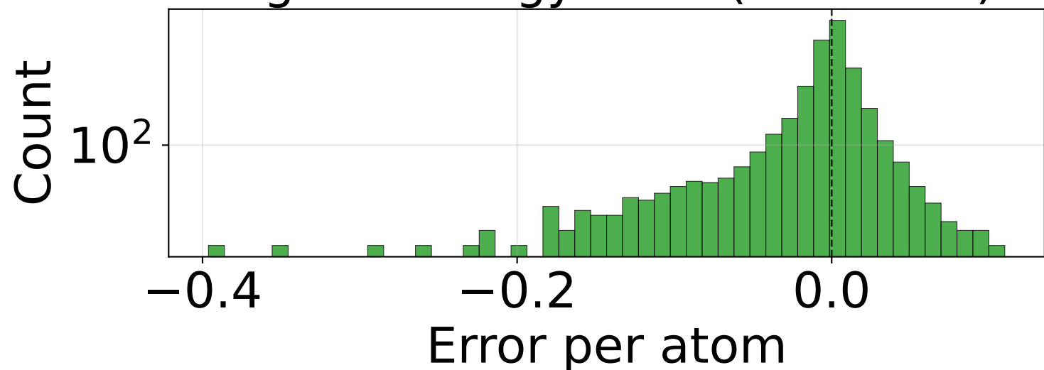
RMSE_E_per_atom (n=49500)
