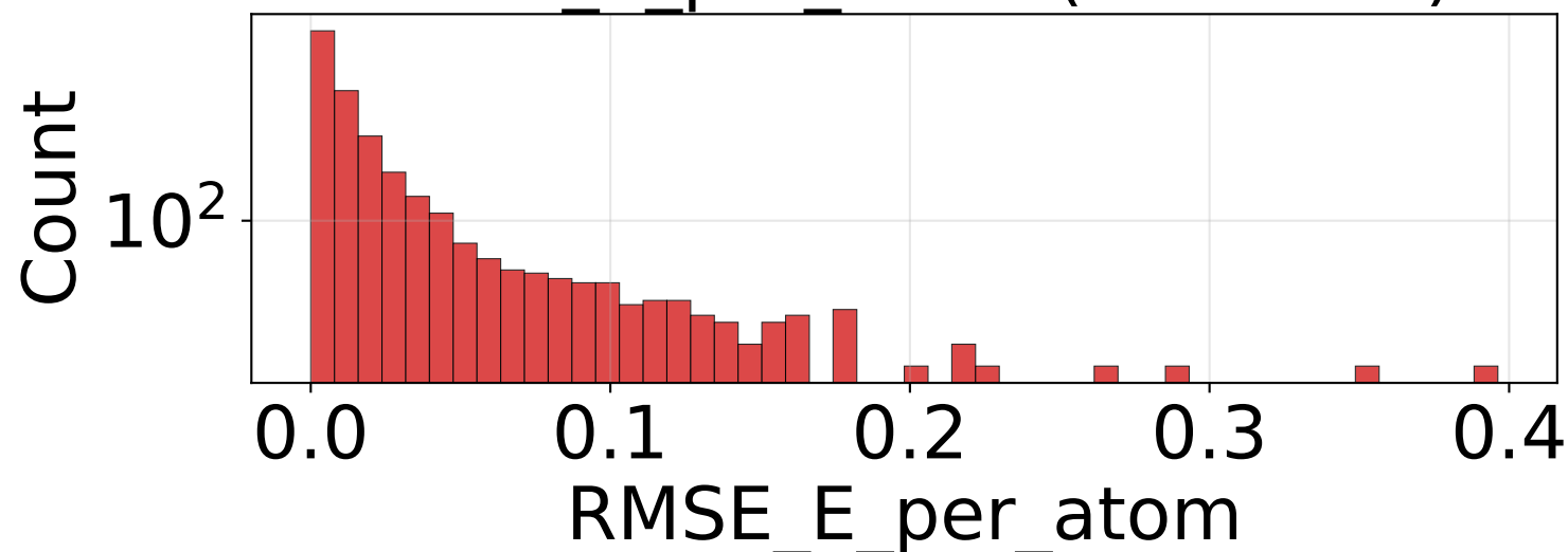
RMSE_E_per_atom (n=49500)
