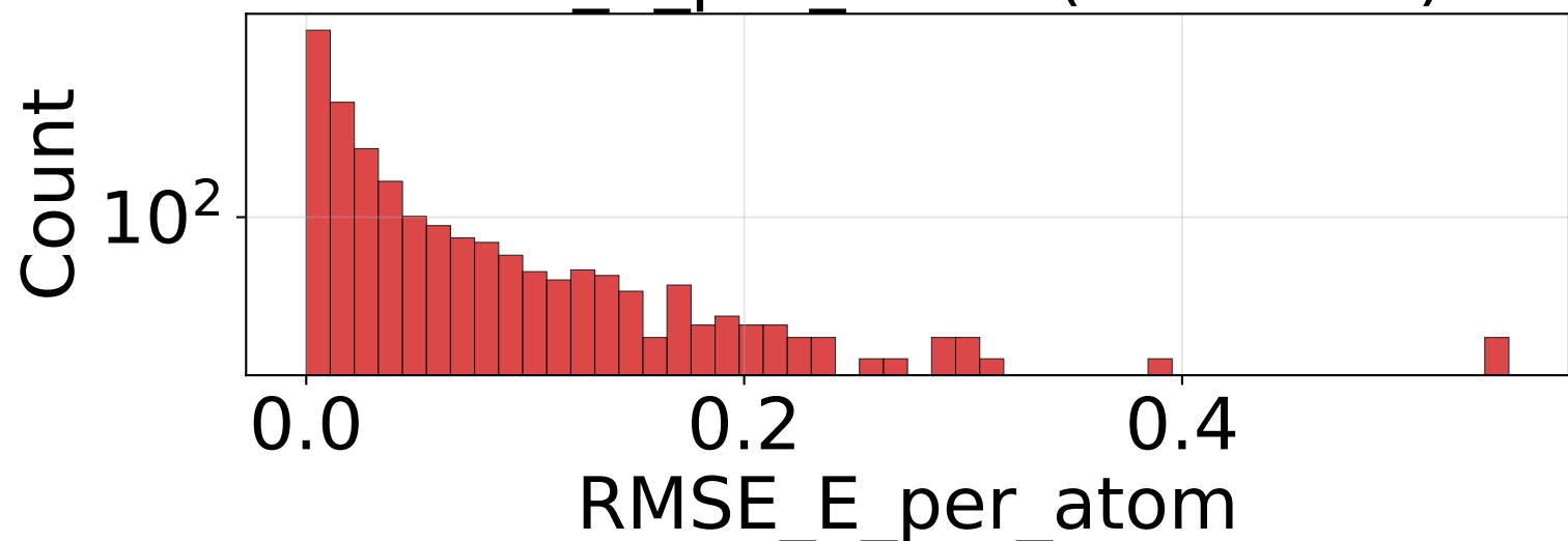
RMSE_E_per_atom (n=49500)
