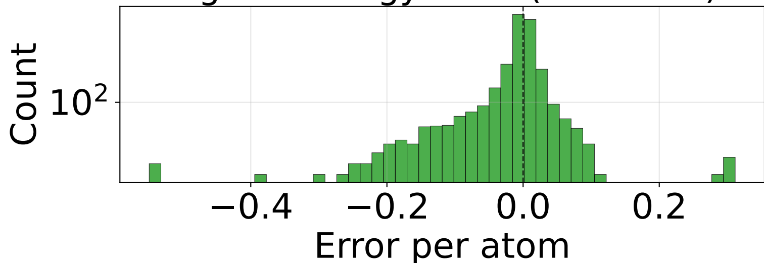
RMSE_E_per_atom (n=49500)
