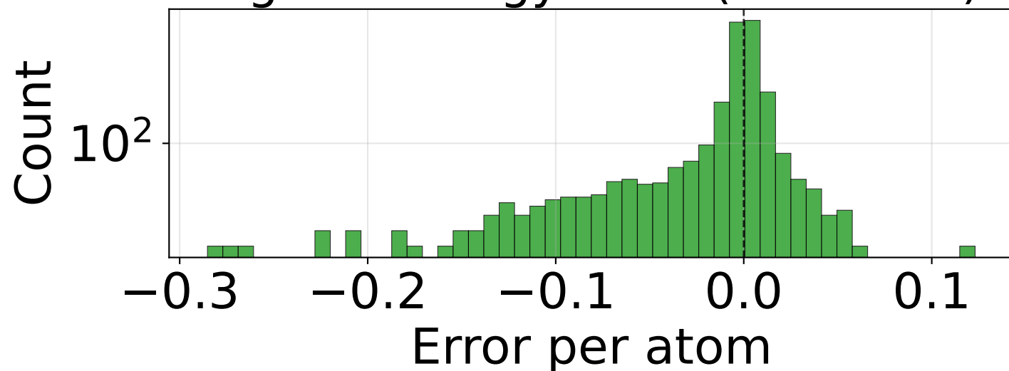
RMSE_E_per_atom (n=49500)
