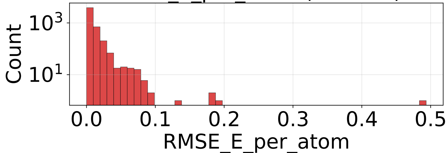
RMSE_E_per_atom (n=4950)
