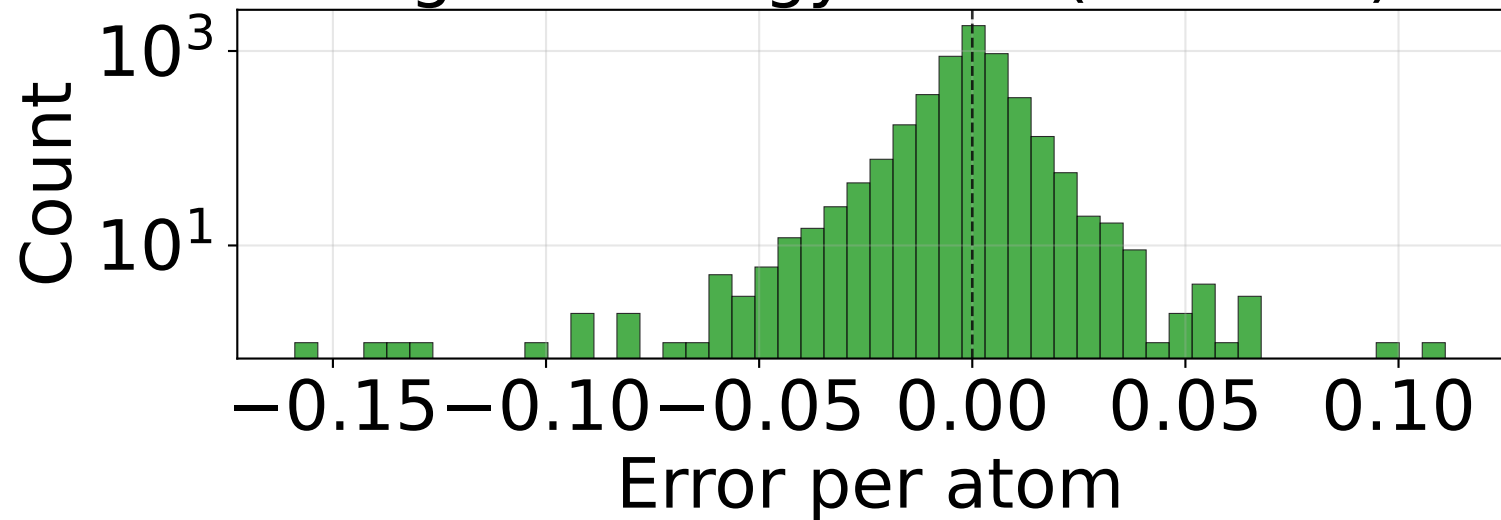
RMSE_E_per_atom (n=4950)
