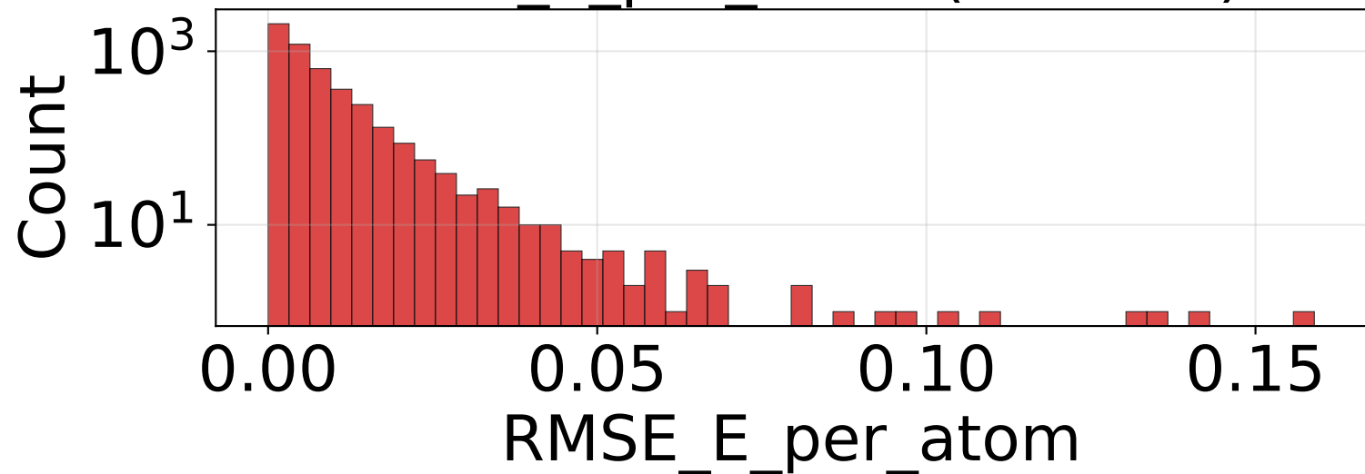
RMSE_E_per_atom (n=4950)
