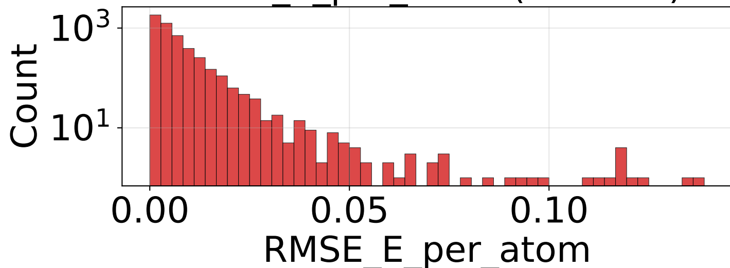
RMSE_E_per_atom (n=4950)
